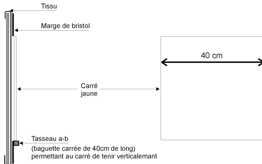
Coupe CD
